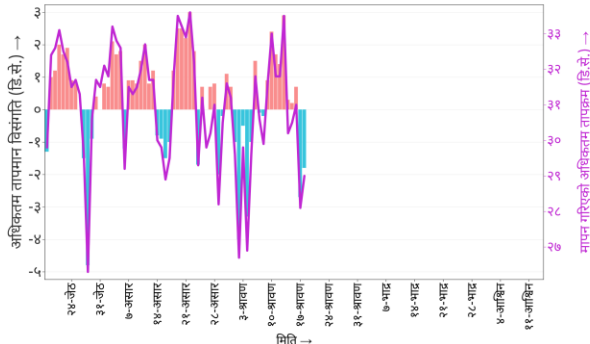
अधिकतम तापक्रम (पोखरा विमानस्थल हवाई मौसम केन्द्र)
