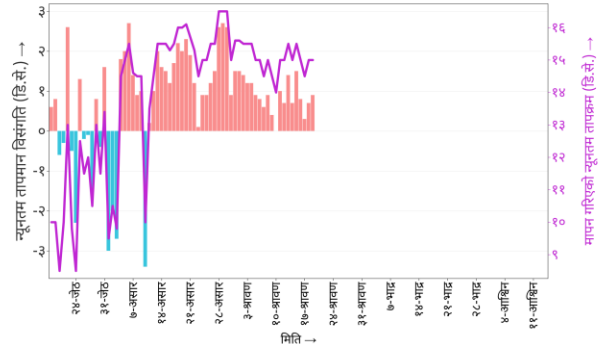
न्यूनतम तापक्रम (जोमसोम एरोसिनटिक केन्द्र)
