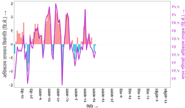
अधिकतम तापक्रम (जोमसोम एरोसिनटिक केन्द्र)
