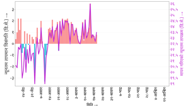
न्यूनतम तापक्रम (पोखरा विमानस्थल हवाई मौसम केन्द्र)
